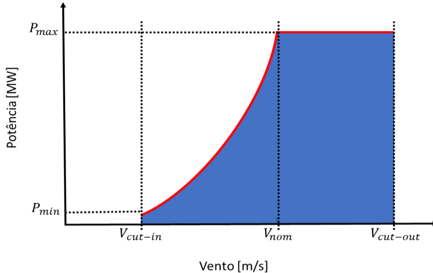
Figura 2 – Representação física da curva Vento x Potência
