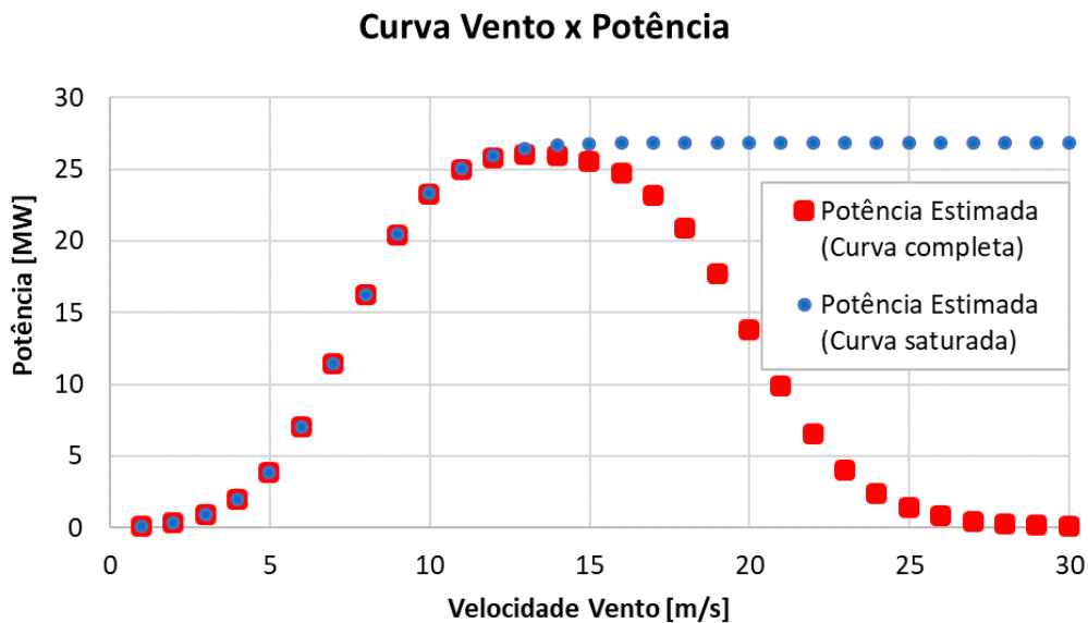
Figura 4 - Curva Vento x Potência com e sem saturação na geração
